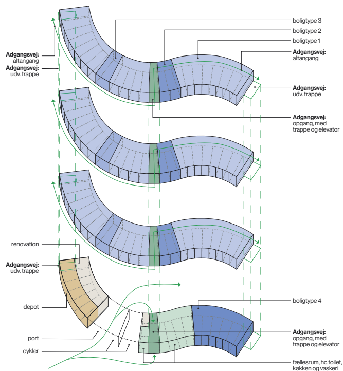
Funktions diagram
